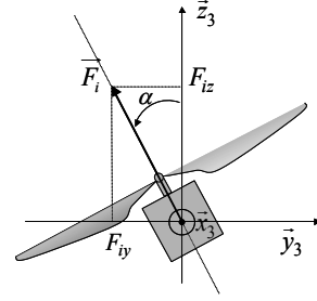
Fig. 8 : Propeller inclination
