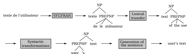
FIG. 1 – SYGFtoE’s architecture
