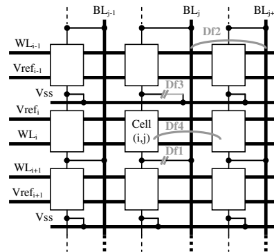
Figure 2.2: Défaits durs dans une matrice eFlash 3*3 bits.
