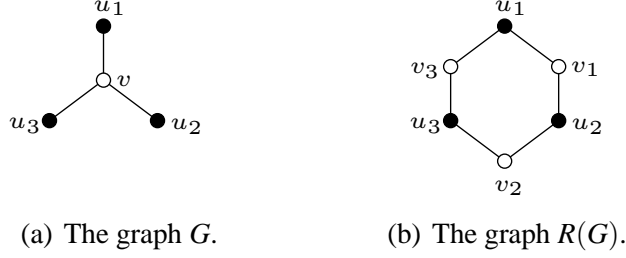
Fig. 4. Configurations of Lemma 13.
