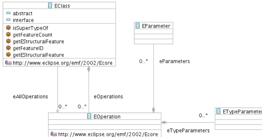
FIG. 5 – Extrait de la partie « EOperation » d'Ecore.
