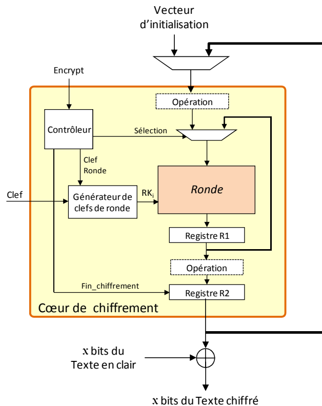
FIGURE 3-2 : MODE DE FONCTIONNEMENT OFB
