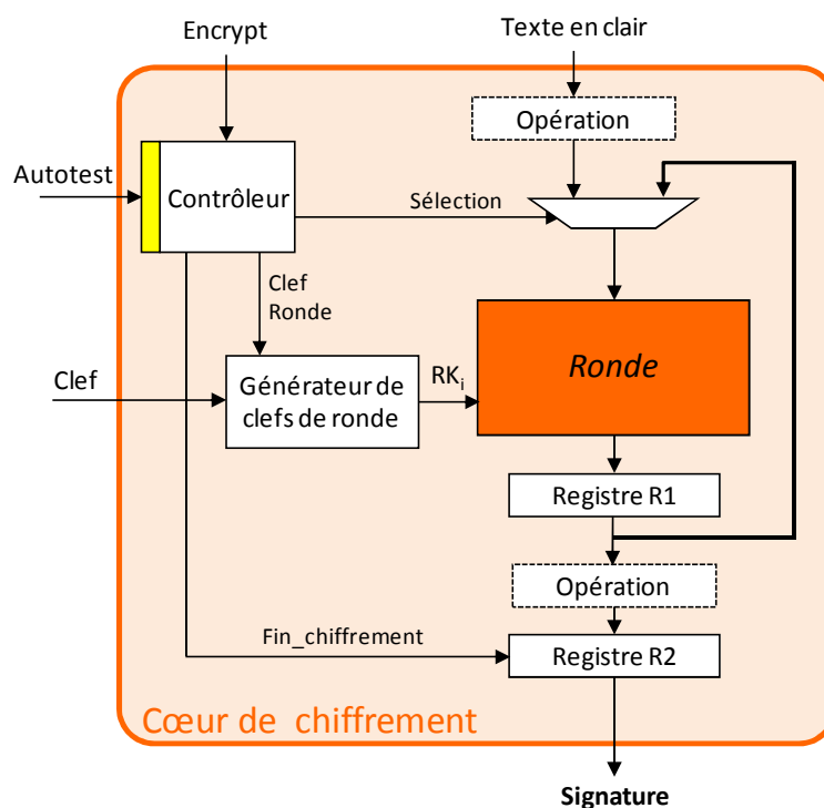
FIGURE 5-1 : MODE AUTOTEST, UTILISANT LA RETROACTION DE RONDE
