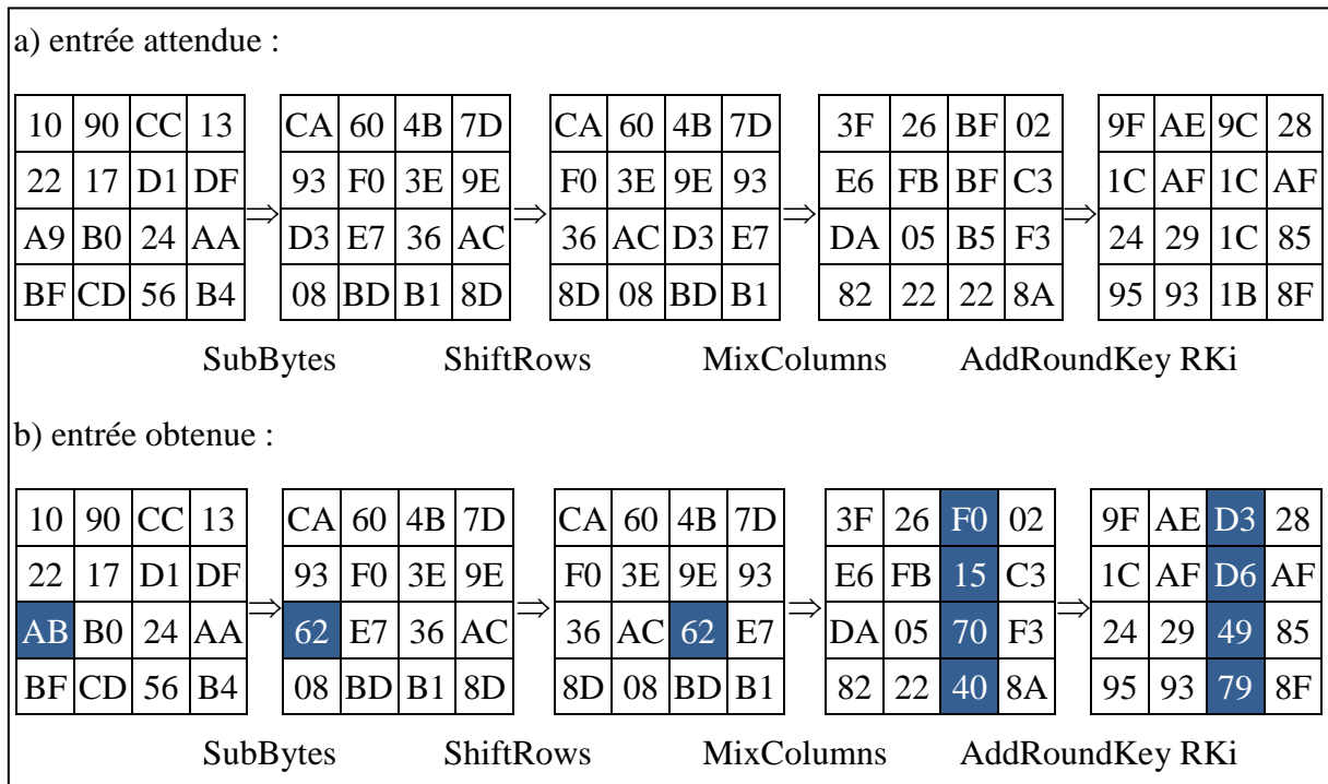
FIGURE 4-9 : PROPAGATION DE L'ERREUR A TRAVERS UNE DES 9 PREMIERES RONDES
