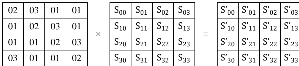
FIGURE 1-9 : PRINCIPE DE L'OPERATION MIX COLUMNS
