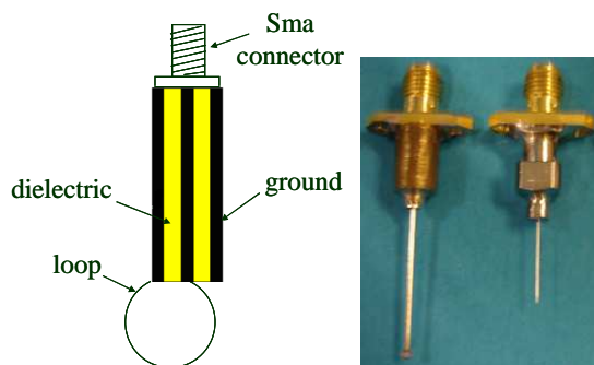
Fig. 22. 500µm and 40µm ØMagnetic probe
