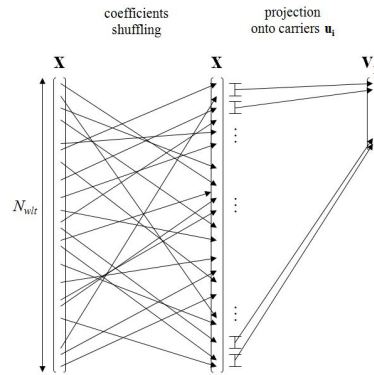
Fig. 5. Random SDM.
