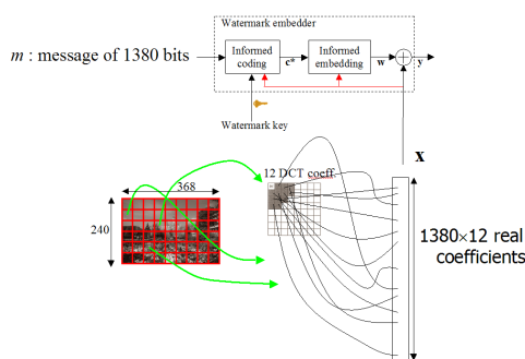
FIGURE 1 – Dirty Paper Trellis Codes appliqués sur une image 240 × 368
