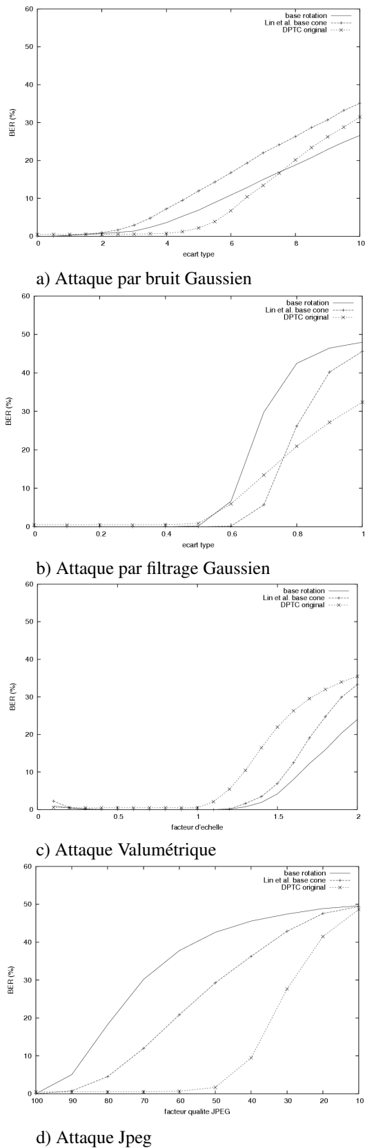
FIGURE 3 – BER pour les attaques sur l’algorithme DPTC original, l’algorithme de Lin et al. basé cône et notre algorithme basé rotation.
