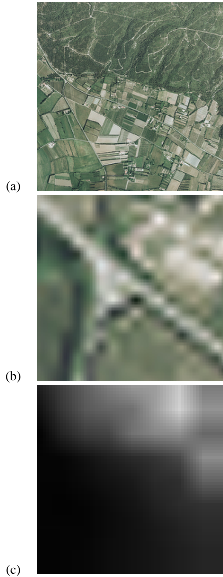
Figure 6 – Reconstruction avec l'image d'approximation du niveau 3 : a) Texture, b) Détail texture, c) Altitudes extraites.
