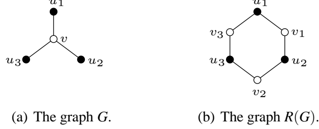
Fig. 4. Configurations of Lemma 13.
