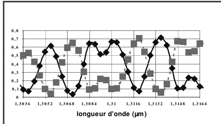
Figure 4 : Spectre [0 1 0 1 1 0 1 0] et complément obtenus en sortie d'un dispositifs WDM avec MMI par regroupement des sorties voisines en utilisant l'entrée 3.
