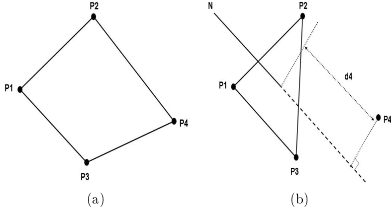
FIG. 5 – a) Quadrangle Q_{1234} , b) Mesure de d_4 pour la contrainte de coplanarité.
