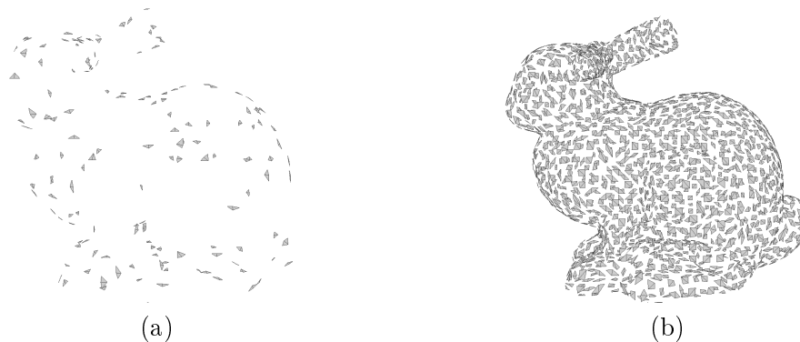
FIG. 14 – Sélection des quadrangles retenus sur le modèle bunny (8146 points, 16301 triangles) avec un seuil S_c de 0.1 : a) 150 quadrangles retenus avec la méthode ACM, b) 1491 quadrangles retenus avec la méthode par projection.
