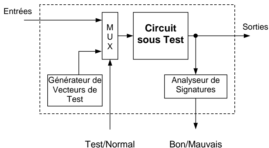
Figure 1 : Schéma de principe du Test Intégré
