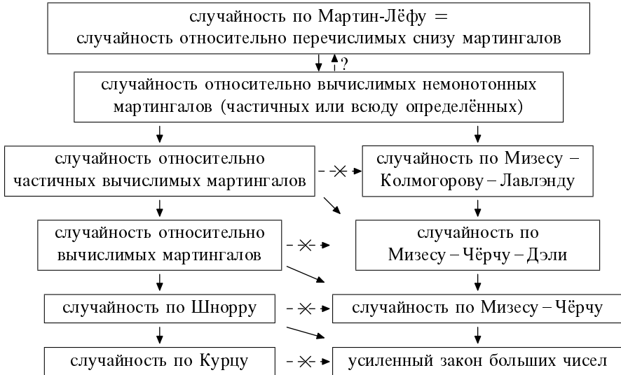
Рис. 9.3. Соотношения между разными определениями случайности.
