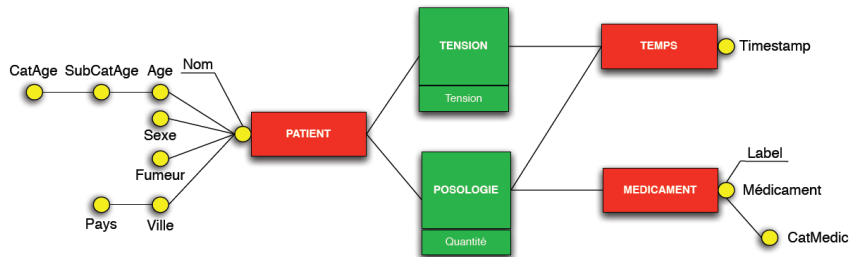
Figure 1. Schéma simplifié de l'entrepôt de données pour l'analyse de la tension et de la posologie
