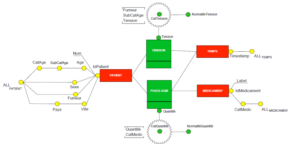
Figure 3. Représentation graphique de l'entrepôt de données médicales
