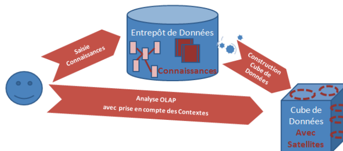
Figure 4. Architecture proposée pour l'exploitation de généralisations de mesures contextualisées
