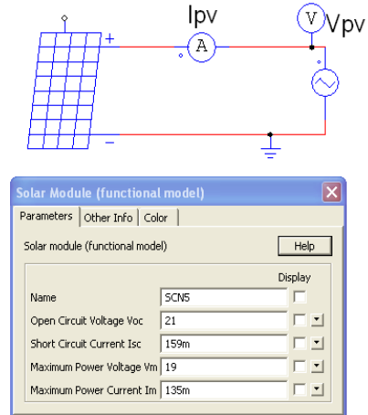
Fig. 12 : Schéma de simulation PSIM et paramétrage du module photovoltaïque.
