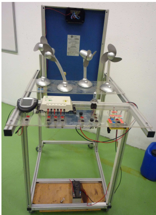
Fig. 10 : Différentes charges et convertisseurs utilisables sur la maquette de Nîmes : hacheur, lampe de phare automobile, moteurs, régulateur de charge de batterie,...
