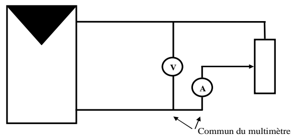
Fig. 6 : Schéma de câble du rhéostat et du multimètre pour relever la caractéristique I(V) du panneau photovoltaïque.
