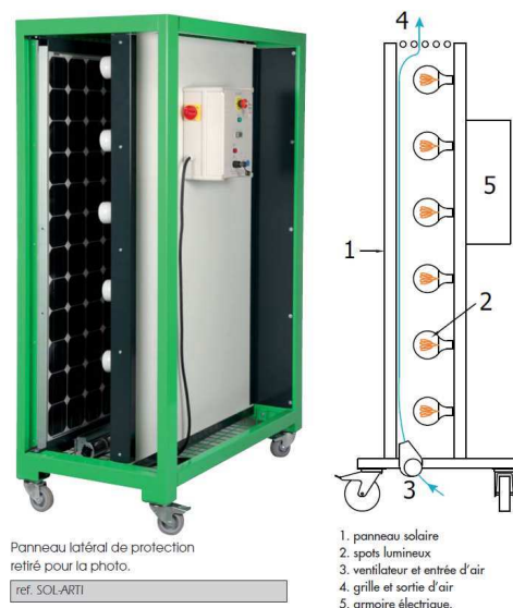
Fig. 15 : La maquette SOL-ARTI proposée par la société LANGLOIS (dimensions : 193 x 123 x 67 cm, poids : 40kg)
