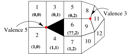
Figure 6: D composition en "polygones rectilignes" : probl me d'ambigu t  sur le positionnement des quadrangles 6 et 11.
