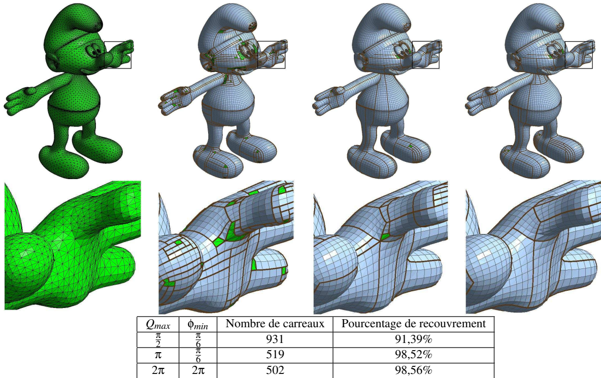
Figure 14: Maillage Schtroumpf avec un zoom et les r sultats obtenus avec Q_{max} = \frac{\pi}{2}, \pi et 2\pi (de gauche   droite). Le nombre de carreaux diminue et leur taille s'accro t. Le recouvrement par la d composition en carreaux s'am liore donc sur cet exemple.
