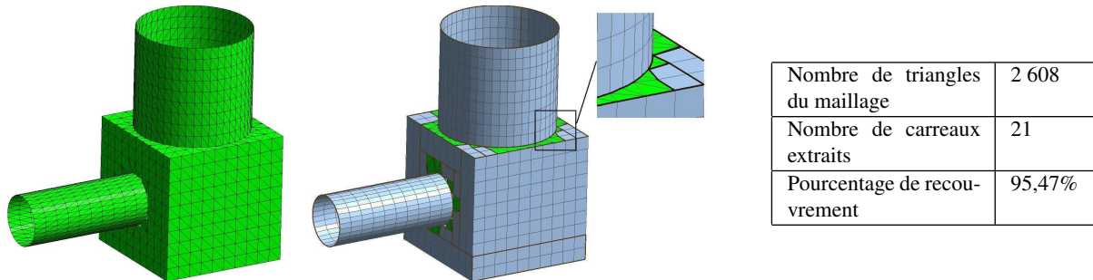
Figure 15: Maillage de d part et r sultat pour : CubeCylindres.
