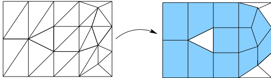
Figure 4: Extraction d'une zone quadrangulée (carreaux pleins) à partir d'un maillage triangulaire. Les triangles restants ne permettent pas de construire des quadrangles de qualité satisfaisante.
