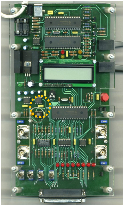
Fig. 3. Maquette de travaux pratiques. Le PIC 18F452 est au centre. A sa gauche, entouré de pointillés jaunes, on voit le capteur de température Maxim Integrated DS 1621.
