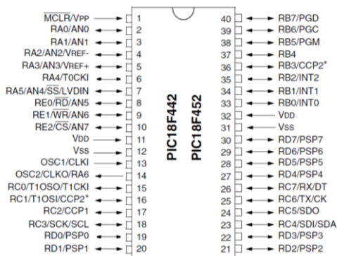
Fig. 1. Brochage du microcontrôleur Microchip PIC 18F452 (extrait de la datasheet du composant).
