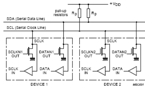
Fig. 4. Support physique du bus I2C (extrait des spécifications Philips [4])
