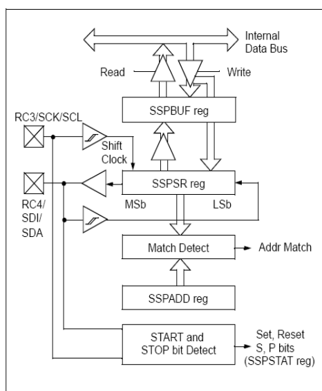
Fig. 7. Schéma du module I2C du PIC18F452 (extrait de la datasheet du composant [1])
