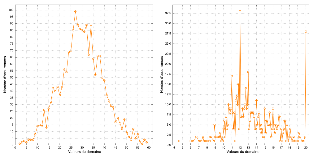
FIG. 5 – Histogramme pour l'attribut var_taxo FIG. 6 – Histogramme pour l'attribut ibd2007
