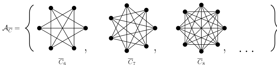
Fig. 3. Antiholes antichain.
