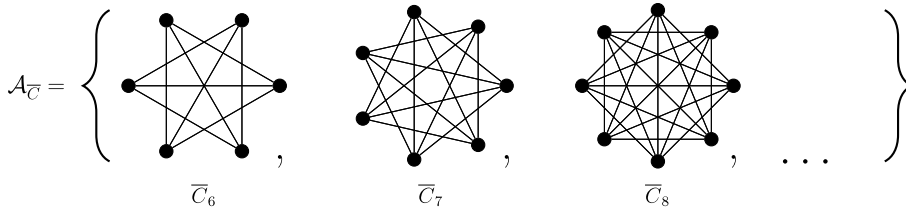
Fig. 3. Antiholes antichain.
