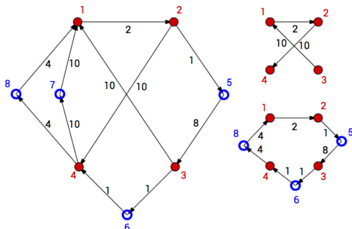
FIGURE 4 – Graphe avec des sommet terminaux en rouge (plein) et potentiels en bleu (cercle). En haut : la solution du MSA sur les sommets terminaux. En bas : la solution au circuit de Steiner sur le graphe entier.
