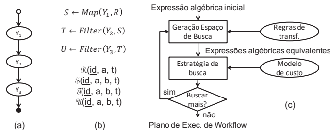
Figura 1. Workflow representado em grafo (a), Workflow representado em álgebra de workflows (b), Processo de otimização de execução de workflows (c)
