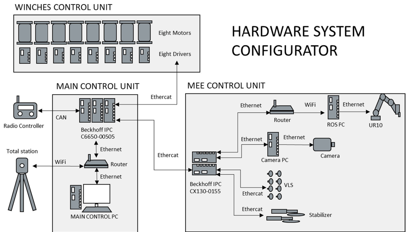
Fig. 22. Hephaestus wiring layout.
