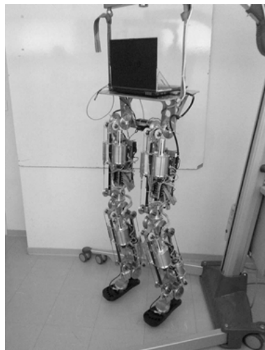
Fig. 3. The SHERPA robot.
