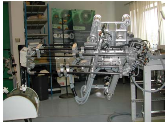
FIG. 14 - Le prototype EndoXirob
