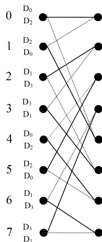
FIGURE 5.1 – La structure du treillis utilisé dans JPEG2000.
