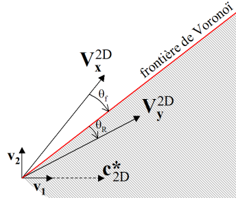
FIGURE 2.3 – Insertion basée rotation dans le plan de Miller, Cox et Bloom
