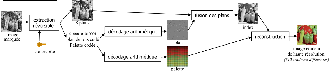
FIGURE 9.1 – Schéma général de l’insertion et de l’extraction pour l’approche de dissimulation par palette de 512 couleurs.
