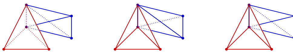
FIGURE 11.11 – Les autres orientations possibles [-, +] , [+, -] et [+, +] (de gauche à droite), correspondant à des crânes n'appartenant pas à la classe BCS.
