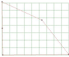
(a) Configuration de points qui est la configuration moyenne des configurations de la Figure 1.2.
