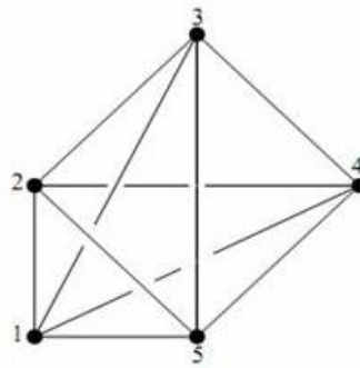
FIGURE 2.1 – Exemple de 5 points en 3 dimensions
