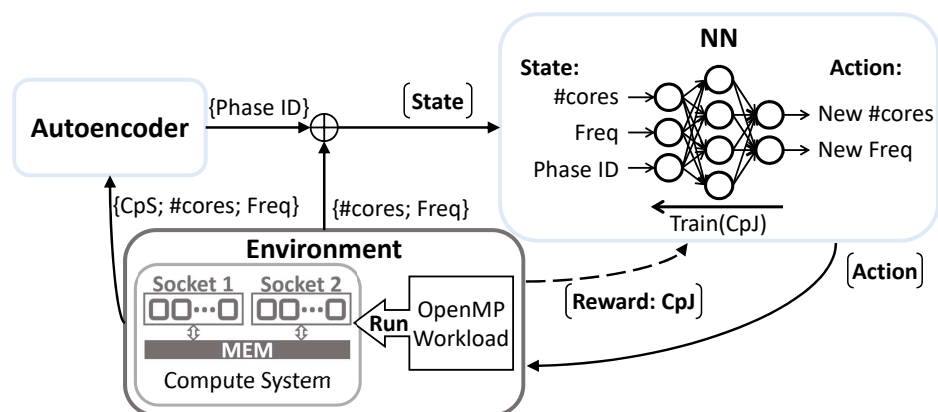
FIGURE 4.17 Système de contrôle avec l'auto-encodeur.
